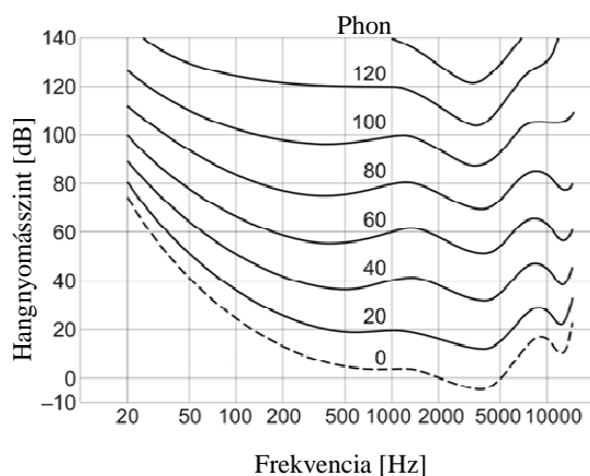
8.2 ábra: Azonos hangosságú szintű görbék
