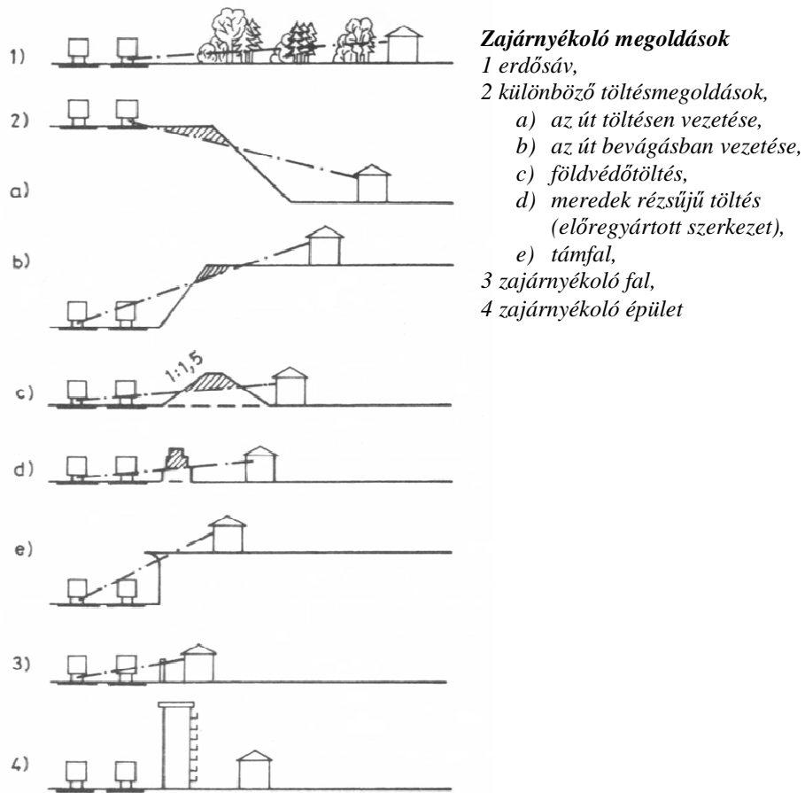
8.10 ábra: Zajárnyékoló falak kialakítási lehetőségei 2.
