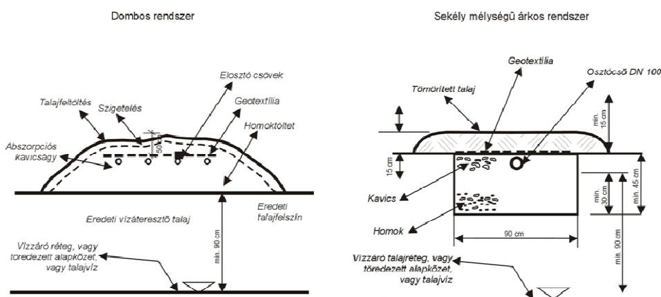
6.7 ábra: Dombos és sekély mélységű árkos szikkasztómező kialakítási sémája
