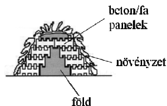
„Bio”-falak kialakítási lehetőségei
