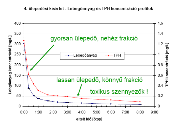
4.13 ábra: Ülepítés vizsgálata (Budai, 2008)
