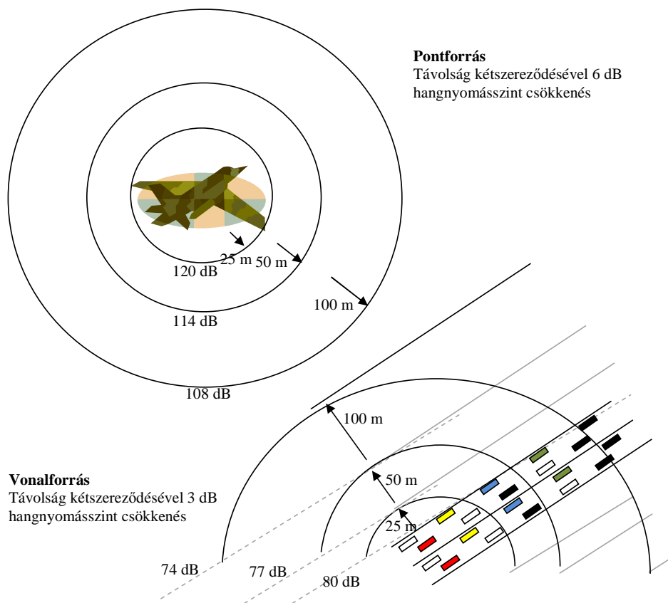
8.7 ábra: Zajcsökkentés mértéke pont- és vonalforrás esetén
