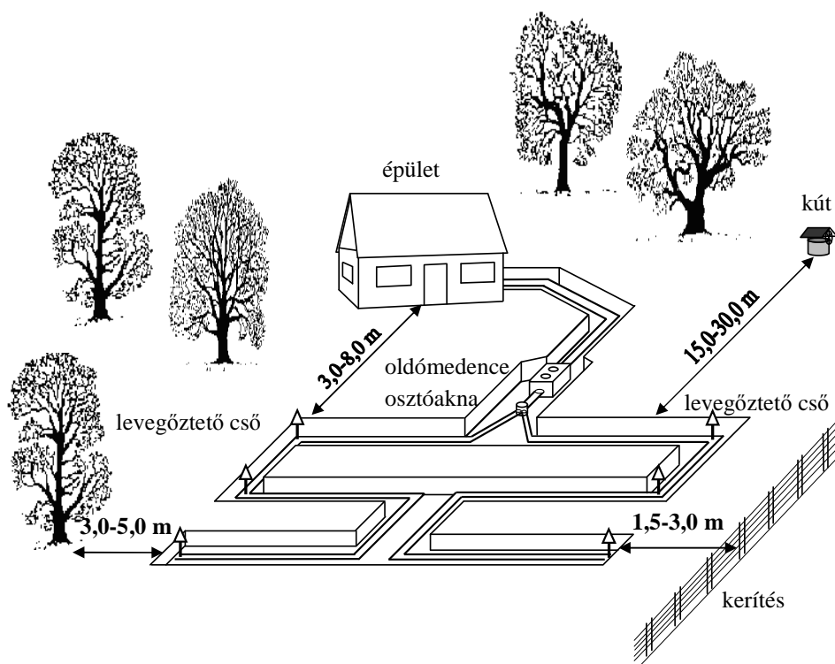
6.8 ábra: Védőtávolságok a szűrőmező kialakításánál
