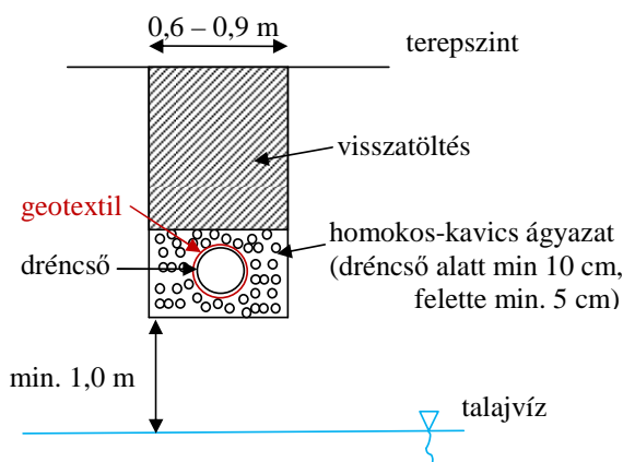
6.6 ábra: A dréncső és az ágyazat keresztmetszete
