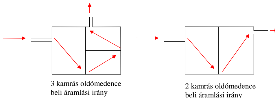
6.3 ábra: Két és háromkamrás oldómedence sematikus
