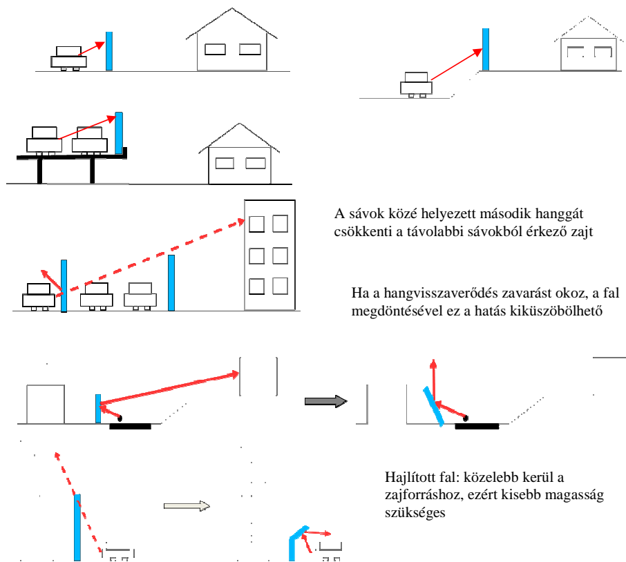
8.9 ábra: Zajárnyékoló falak kialakítási lehetőségei 1.
