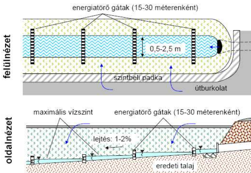
4. 10 ábra: Füvesített vízvezető árok (Claytor és Schueler, 1996)
