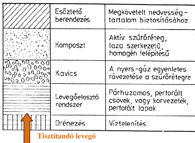
3.5 ábra: Komposztiszűrő elvi sémája
