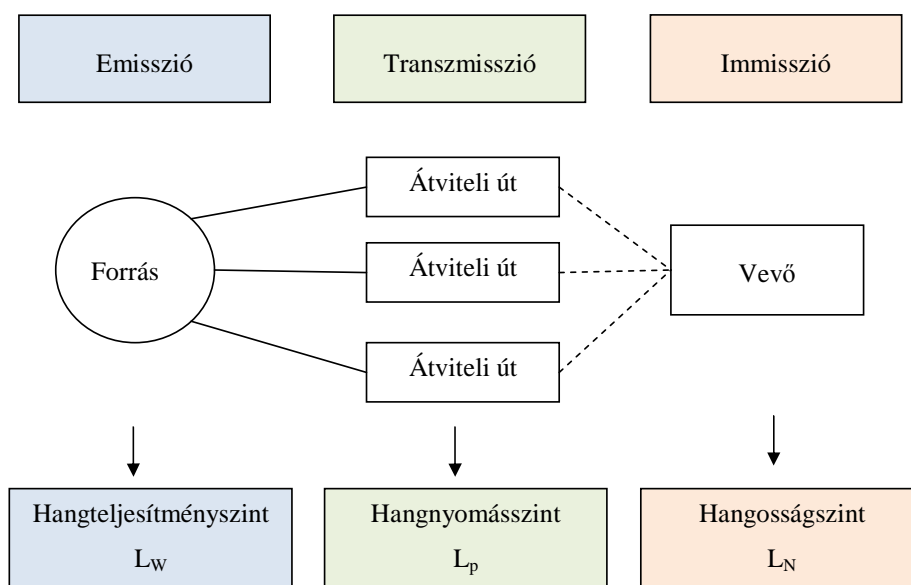
8.8 ábra: Zajcsökkentési lehetőségek helyei
