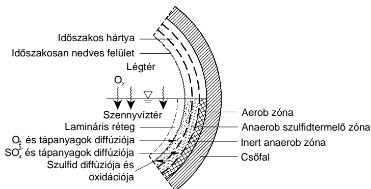
3.1 ábra: Biológiai hártya
