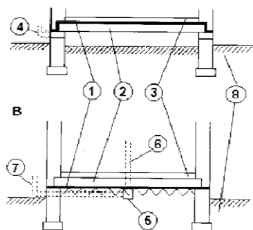
8.13 ábra: Radongátak elhelyezési lehetőségei
