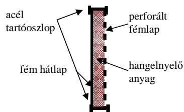
Fémszerkezetű zajvédő fal
