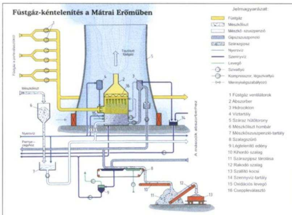
2.1 ábra: A Mátrai Erőmű füstgázának kéntelenítő mosótornya
