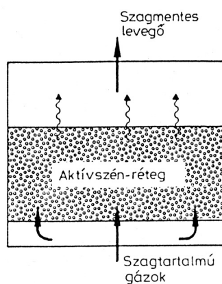
3.4 ábra: Adszorpciós biofilter elvi ábrája
