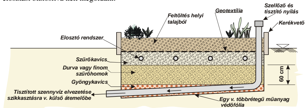
6.5 ábra: Homokszűrő kialakítása
