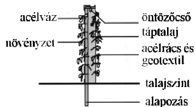
8.11 ábra: Zajvédő falak anyaguk szerint
