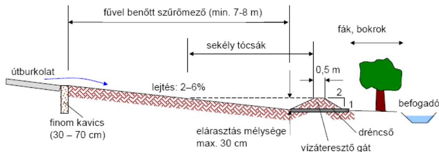
4.11 ábra: Pufferzóna kialakítása
